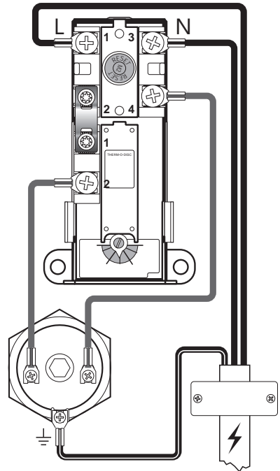
El-kobling, skjematisk
