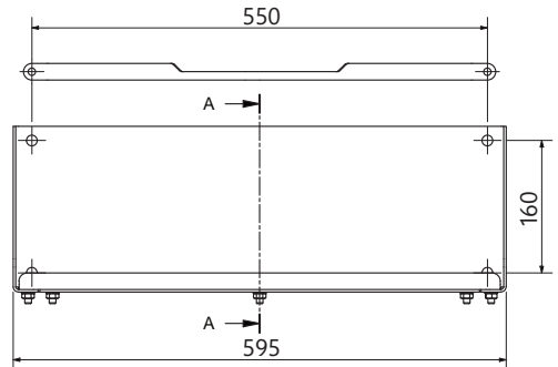
Veggbrakett side
