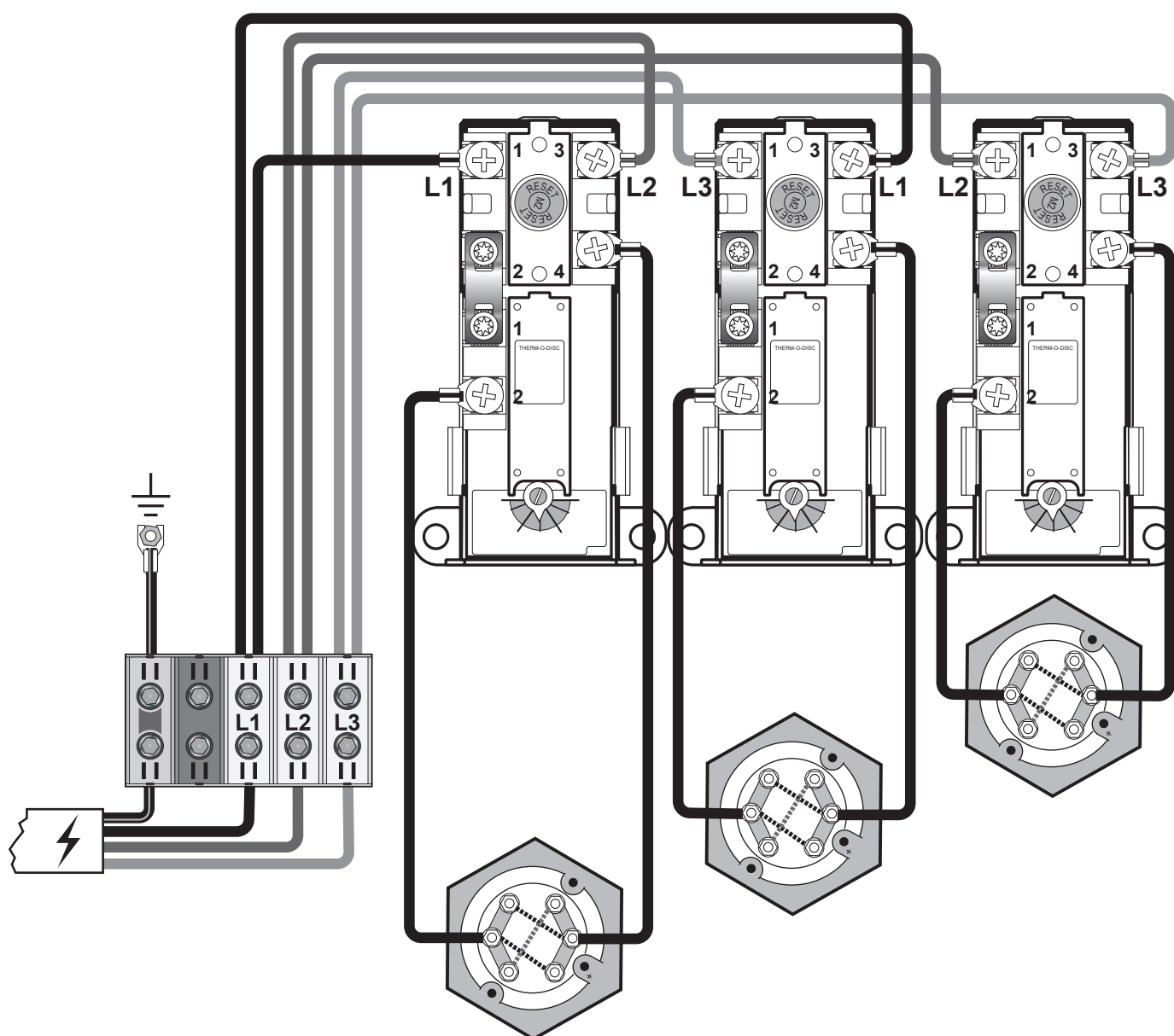
Skjematisk el-kobling 15 kW (3x5kW, 3-rørs elementer) - 3-fas 230V
