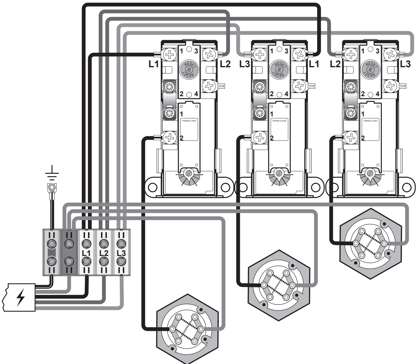
Skjematisk el-kobling 15 kW (3x5kW, 3-rørs elementer) - 3-fas 400V med nulleleder
