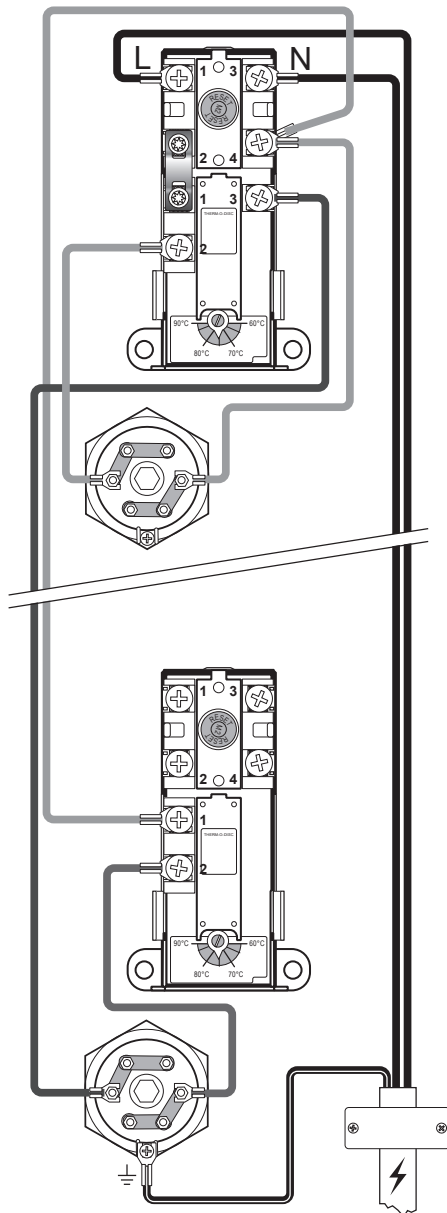
EI-kobling skjematisk - 4,5+4,5 kW
