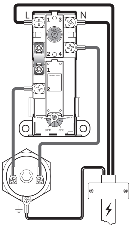
El-kobling, skjematisk
