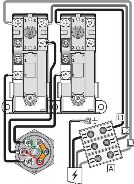
El-kobling, skjematisk - 9 kW - 3x400V Alt. kobl. for nedre magasin - Nulleider kan IKKE benyttes!
