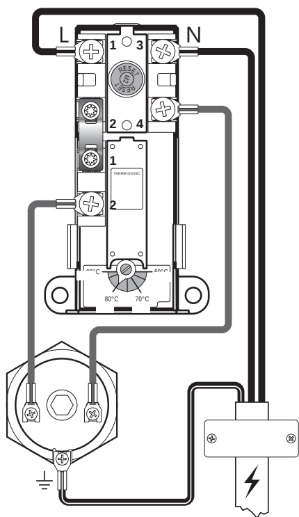
El-kobling, skjematisk
