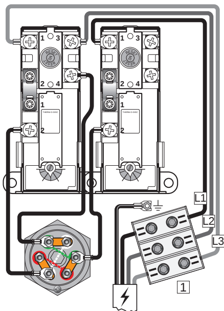
El-kobling, skjematisk - STANDARD 7.5 kW - 230V - 3 - 50Hz Nedre magasin har to identiske el-sentraler.
