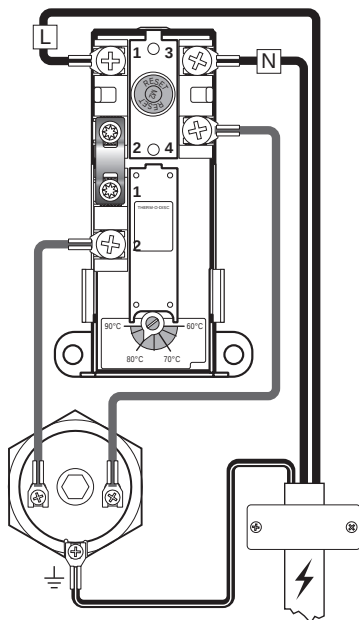
El-kobling, skjematisk - STANDARD 3 kW - 230V - 50Hz Standard kobling for øvre magasin.
