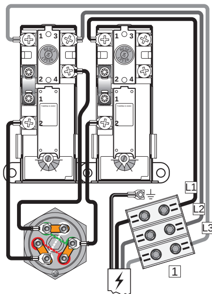
El-kobling, skjematisk - STANDARD 7.5 kW - 230V - 3 - 50Hz Nedre magasin har to identiske el-sentraler.
